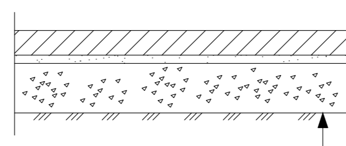
Покриття спортивних майданчиків М1:10
