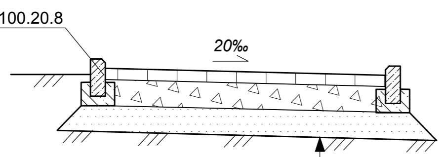
Покриття тротуарів М1:20
